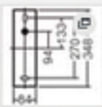
取付図
